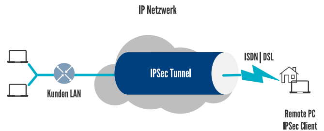
Abb.: Remote Access / Einwahl
